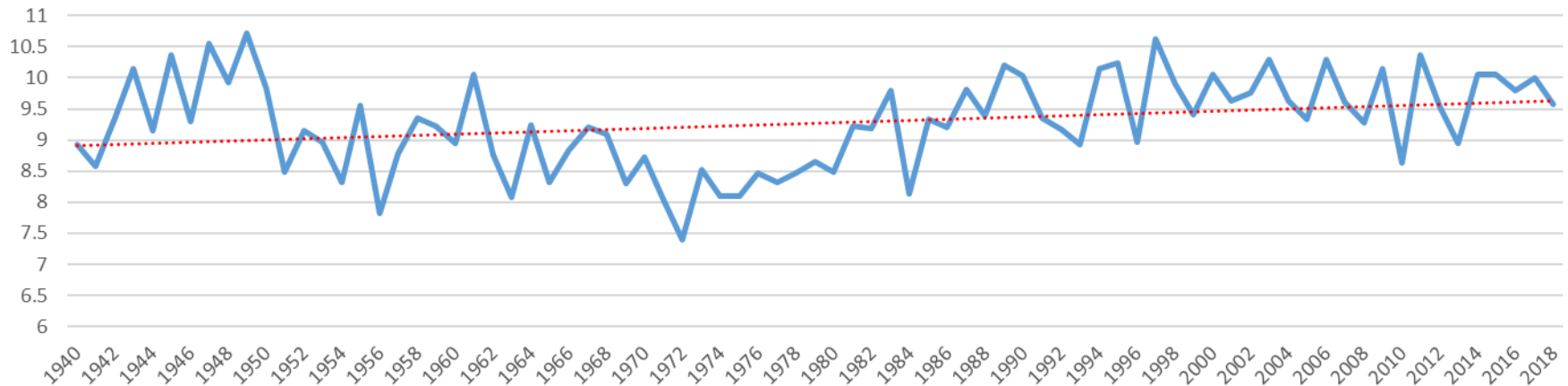
Temperatura media Anual - Aragón (1940 - 2018)
